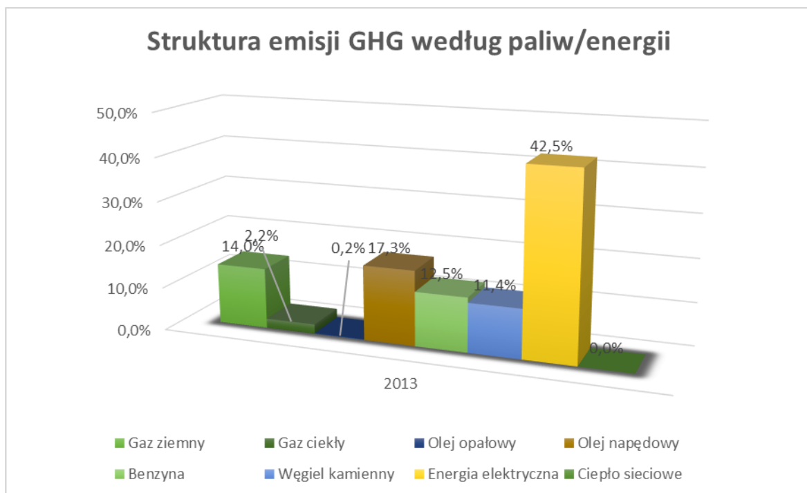
Rysunek 11. Procentowy udział źródeł energii w całkowitej emisji CO 2 z terenu gminy Puszczykowo w 2013 roku
