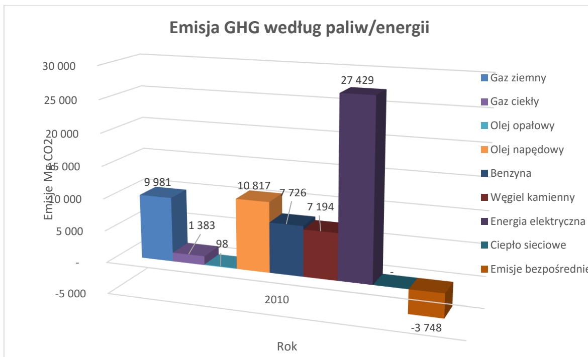
Rysunek 6. Wielkość emisji CO 2 z terenu gminy Puszczykowo w 2010 roku wg źródeł energii Źródło: opracowanie własne
