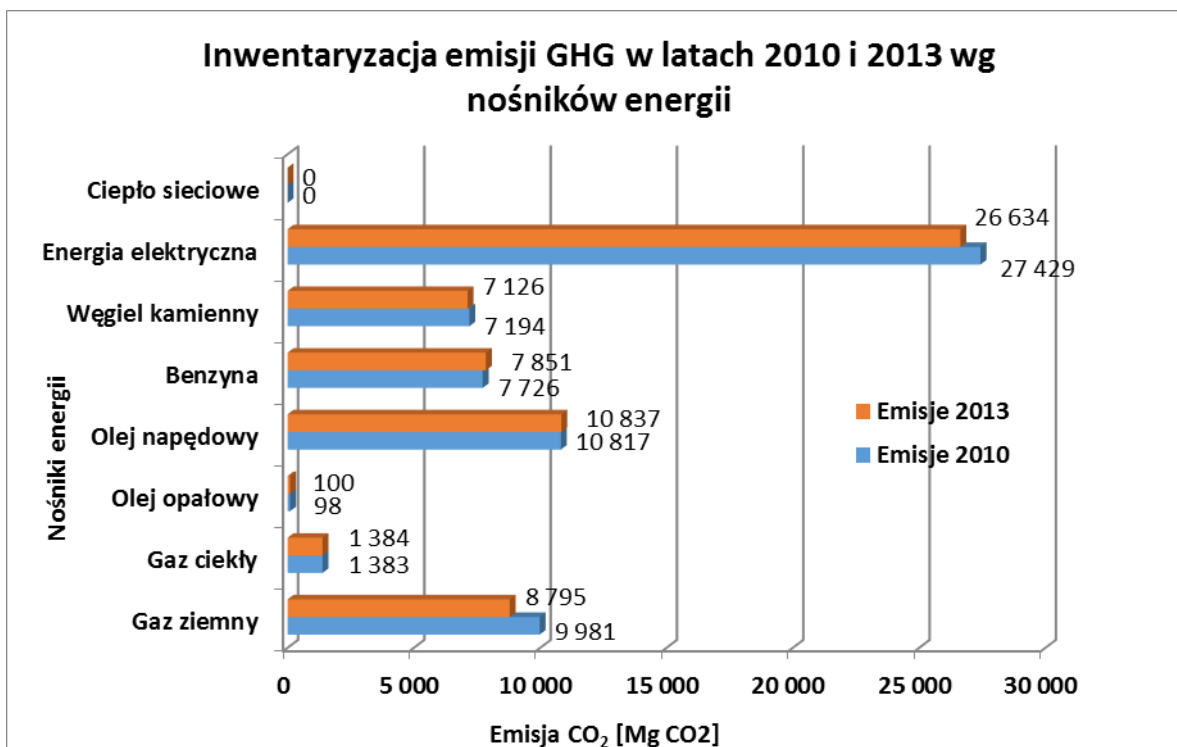
Rysunek 13. Inwentaryzacja emisji GHG w latach 2010 i 2013 w gminie Puszczykowo wg nośników energii
