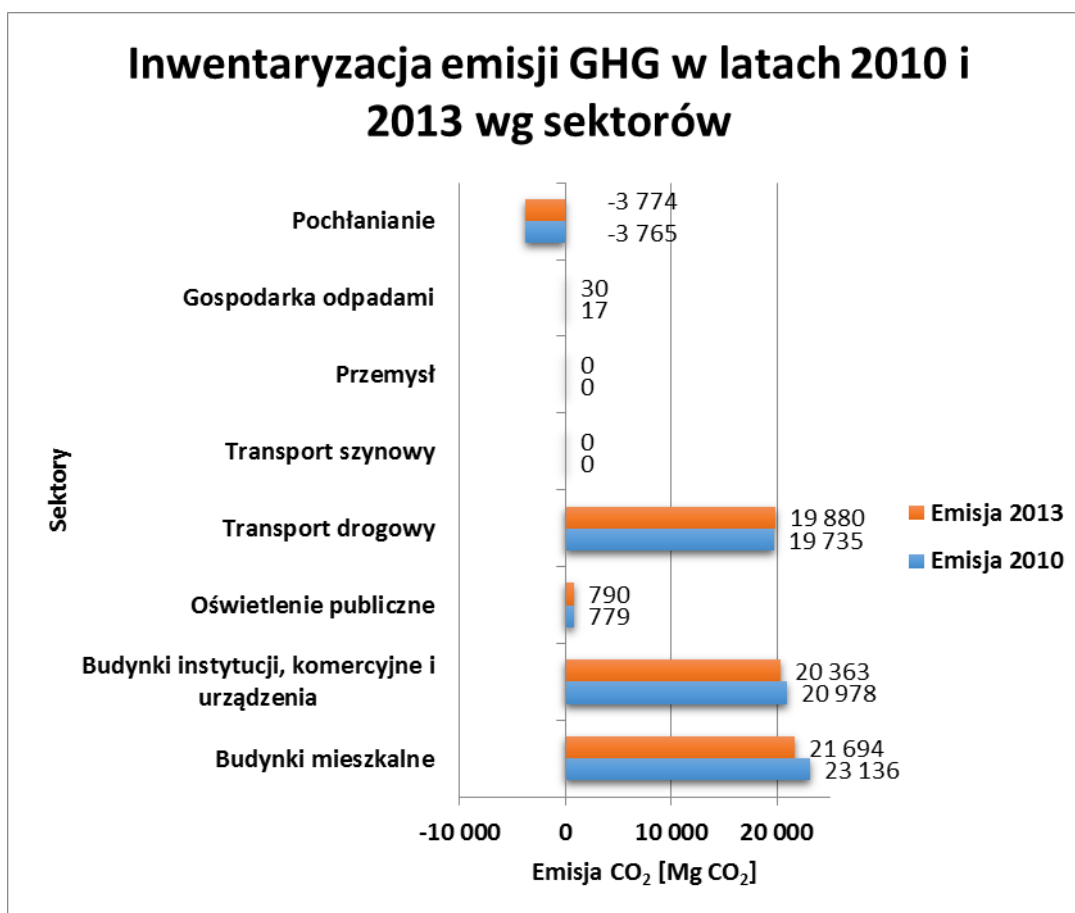
Rysunek 12. Inwentaryzacja emisji GHG w gminie Puszczykowo w latach 2010 i 2013 wg sektorów
