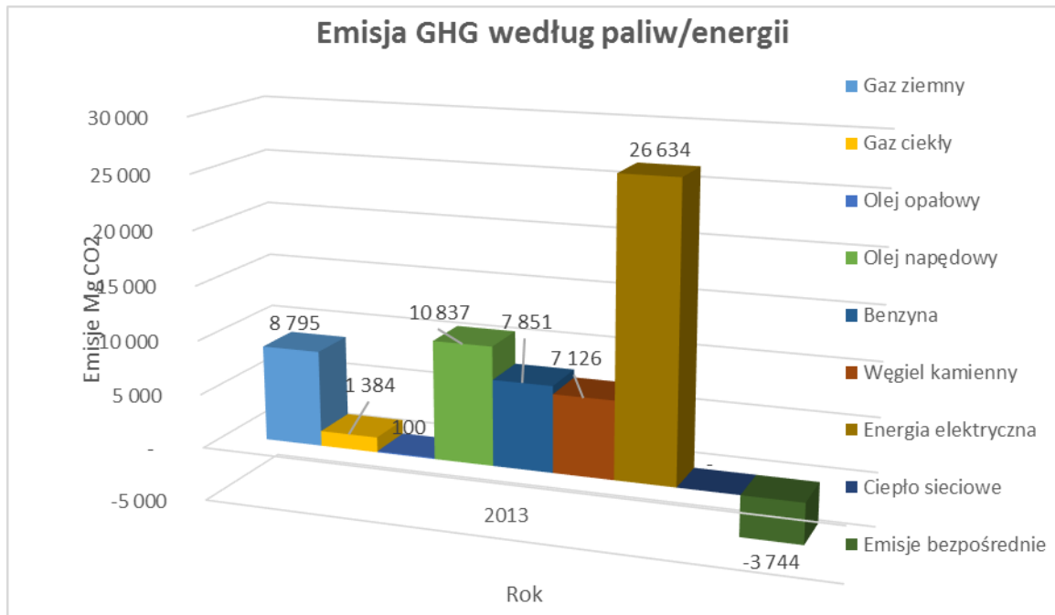
Rysunek 10. Wielkość emisji CO 2 z terenu gminy Puszczykowo w 2013 roku wg źródeł energii Źródło: opracowanie własne
