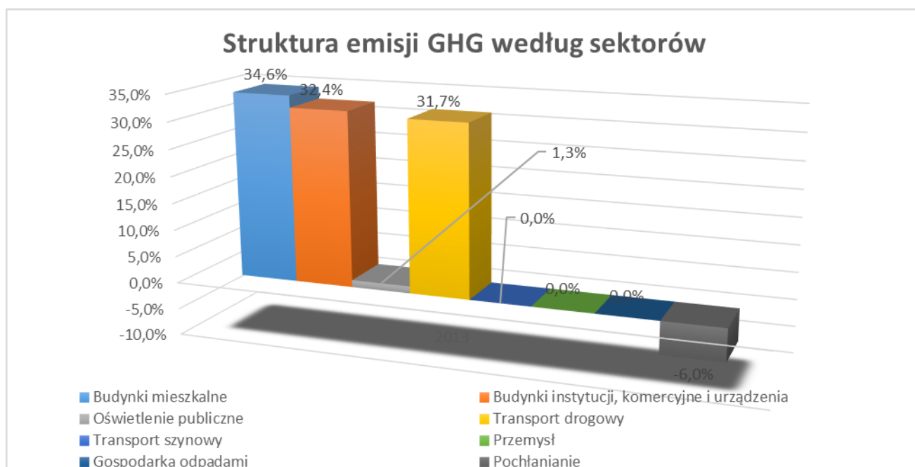
Rysunek 9. Procentowy udział sektorów w całkowitej emisji CO 2 z terenu gminy Puszczykowo w 2013 roku Źródło: opracowanie własne
