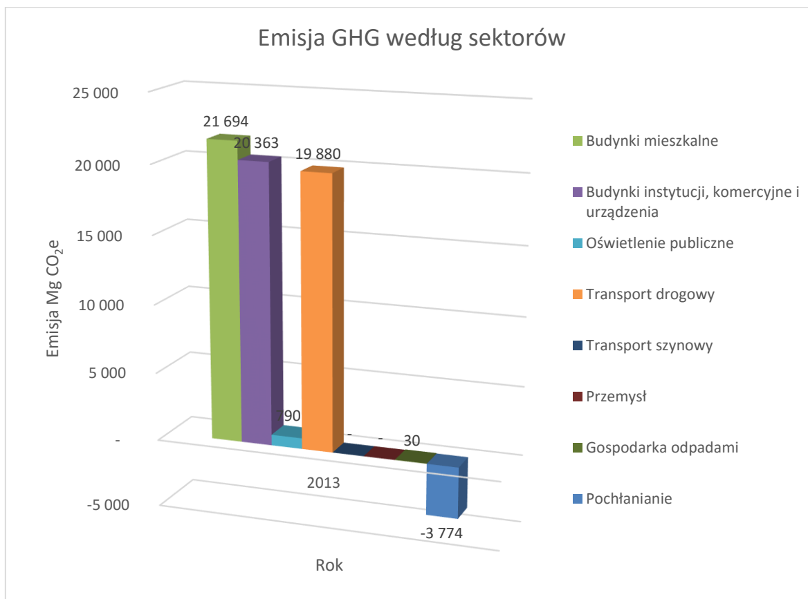
Rysunek 8. Wielkość emisji CO 2 z terenu gminy Puszczykowo w 2013 roku wg sektorów Źródło: opracowanie własne
