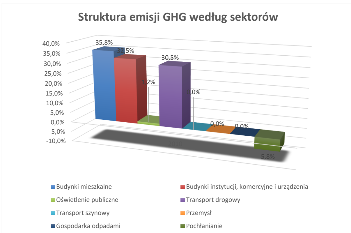
Rysunek 5. Procentowy udział sektorów w całkowitej emisji CO 2 z terenu gminy Puszczykowa w 2010 roku
